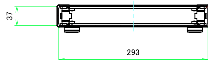
B-B (1 : 4.5)
