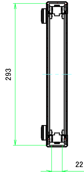
A-A (1 : 4.5)
