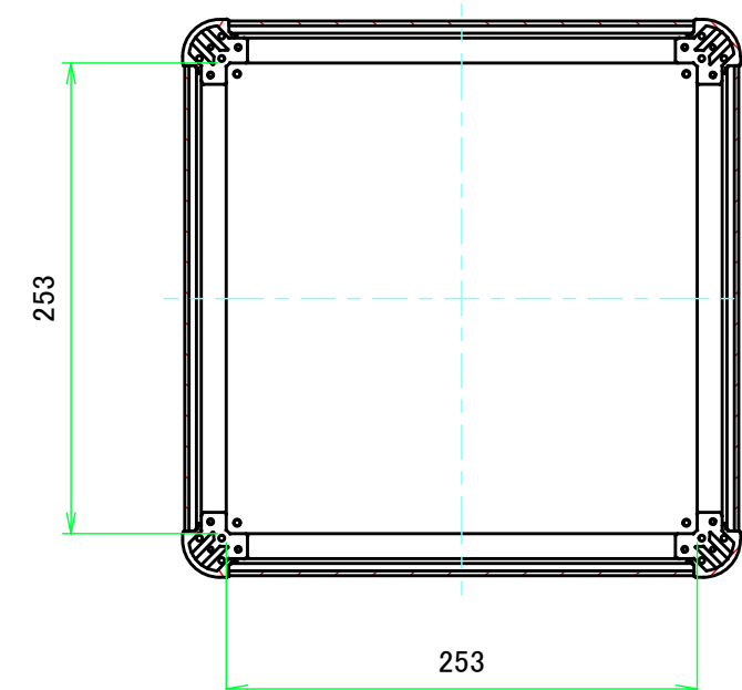
C-C (1 : 4.5)
